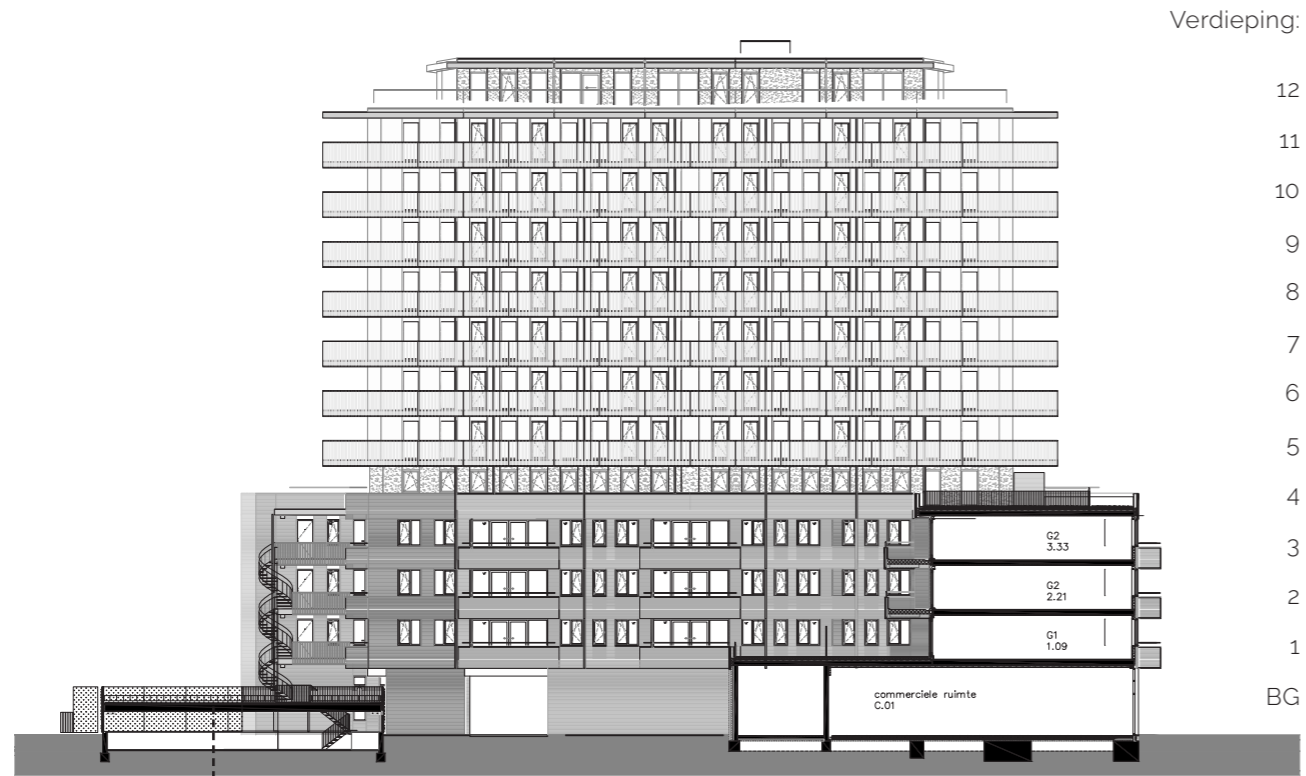
Tweelaagse parkeergelegenheid
